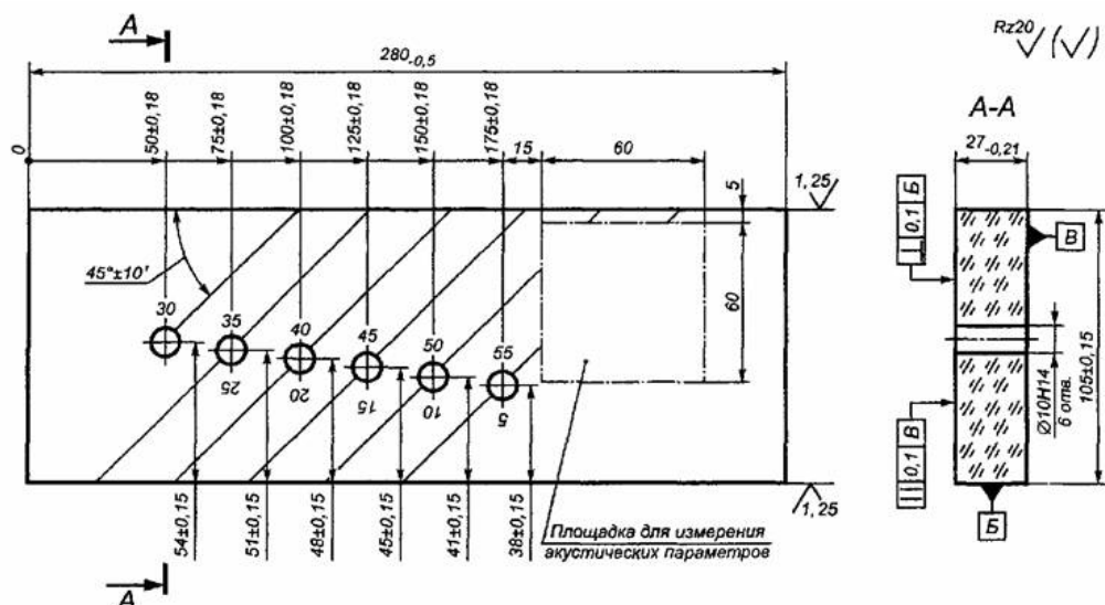
Рисунок 2 — Стандартный образец СО-1Р
