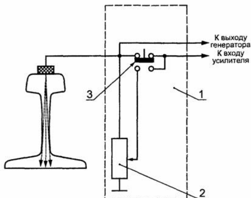
1 - имитатор дефектов; 2 — аттенюатор; 3 - переключатель
