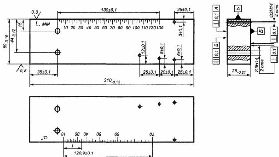
Рисунок 3 — Стандартный образец СО-2Р
