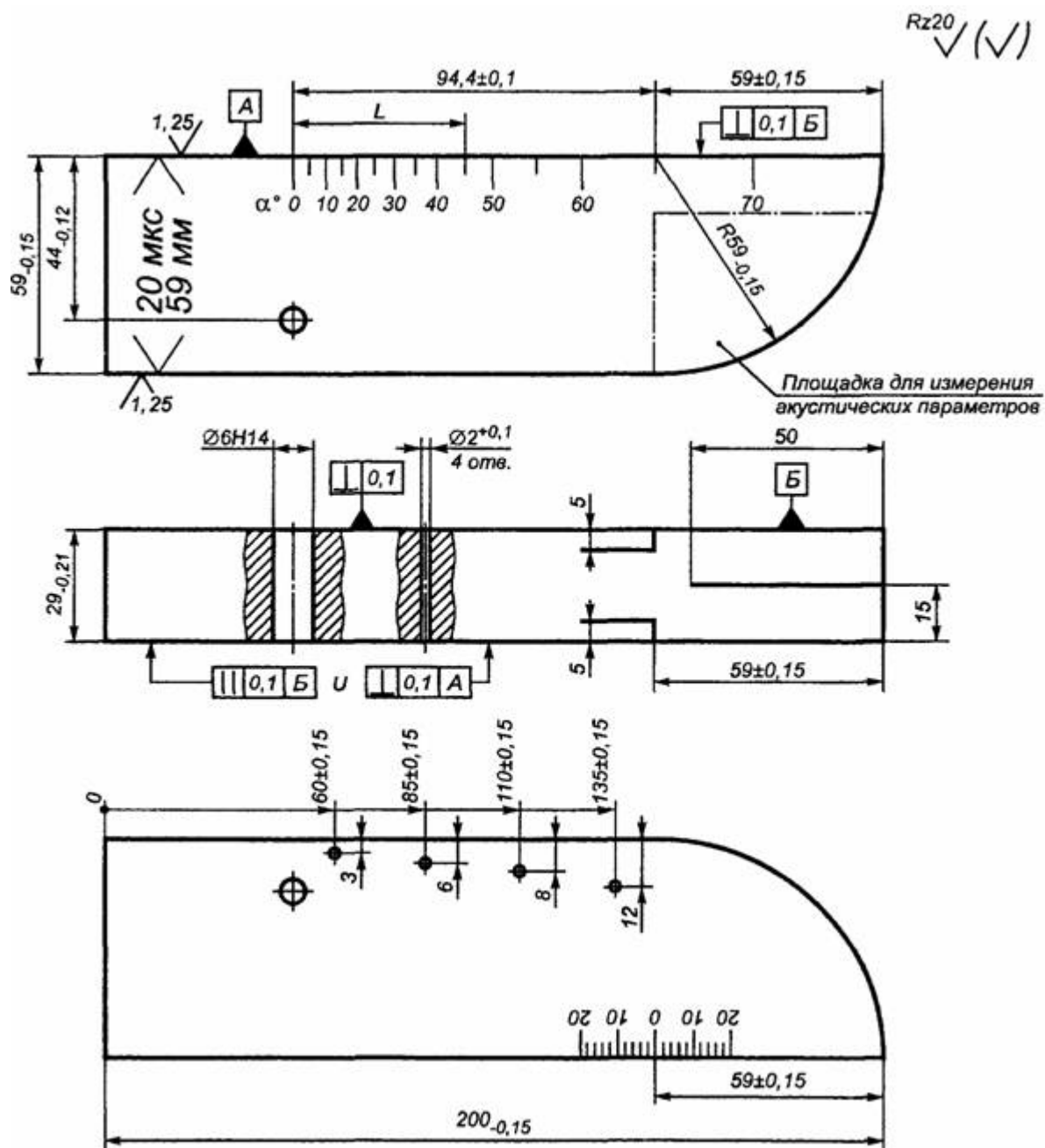
Рисунок 4 — Стандартный образец СО-3Р
