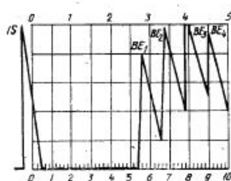
Плохое соединение (преобразователь с двумя кристаллами)
