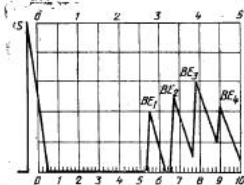
Удовлетворительное соединение (преобразователь с двумя кристаллами)
