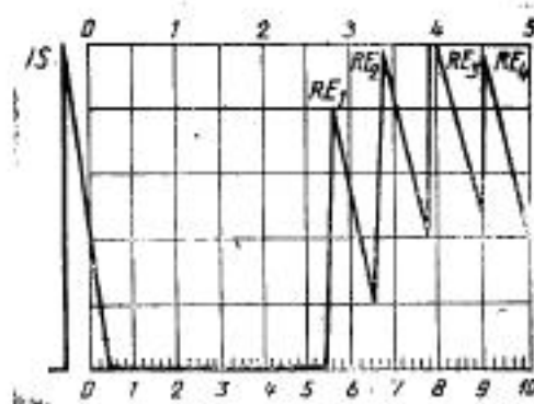
Установление звукового сигнала при помощи преобразователя с двойными кристаллами
