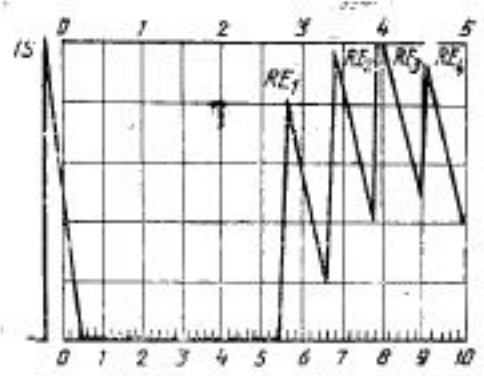
Установление звукового сигнала при помощи преобразователя с двумя кристаллами
