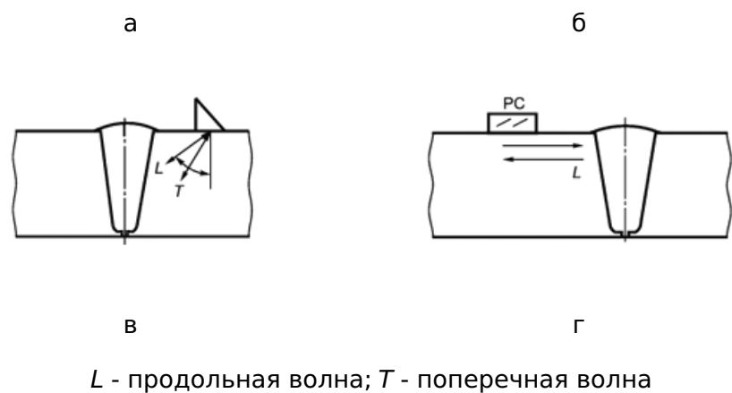
Рисунок 1 - Схемы прозвучивания
