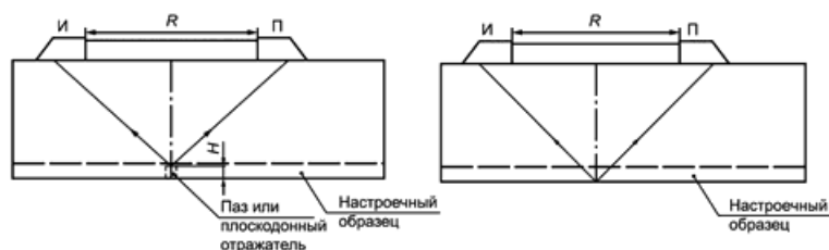
б) Схема настройки дефектоскопа
