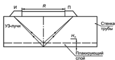
а) Схема измерения
